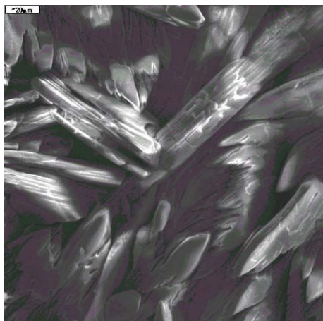
SURFACOTE 480, 500-szoros nagyítás
