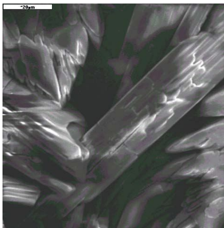
SURFACOTE 480, 1000-szoros nagyítás
