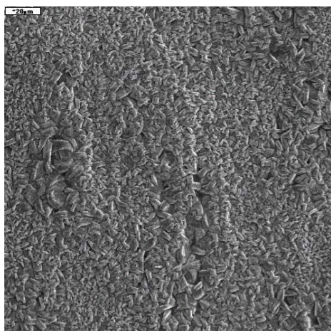
SURFACOTE 775, 500-szoros nagyítás
