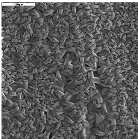
SURFACOTE 775, 1000-szeres nagyítás
